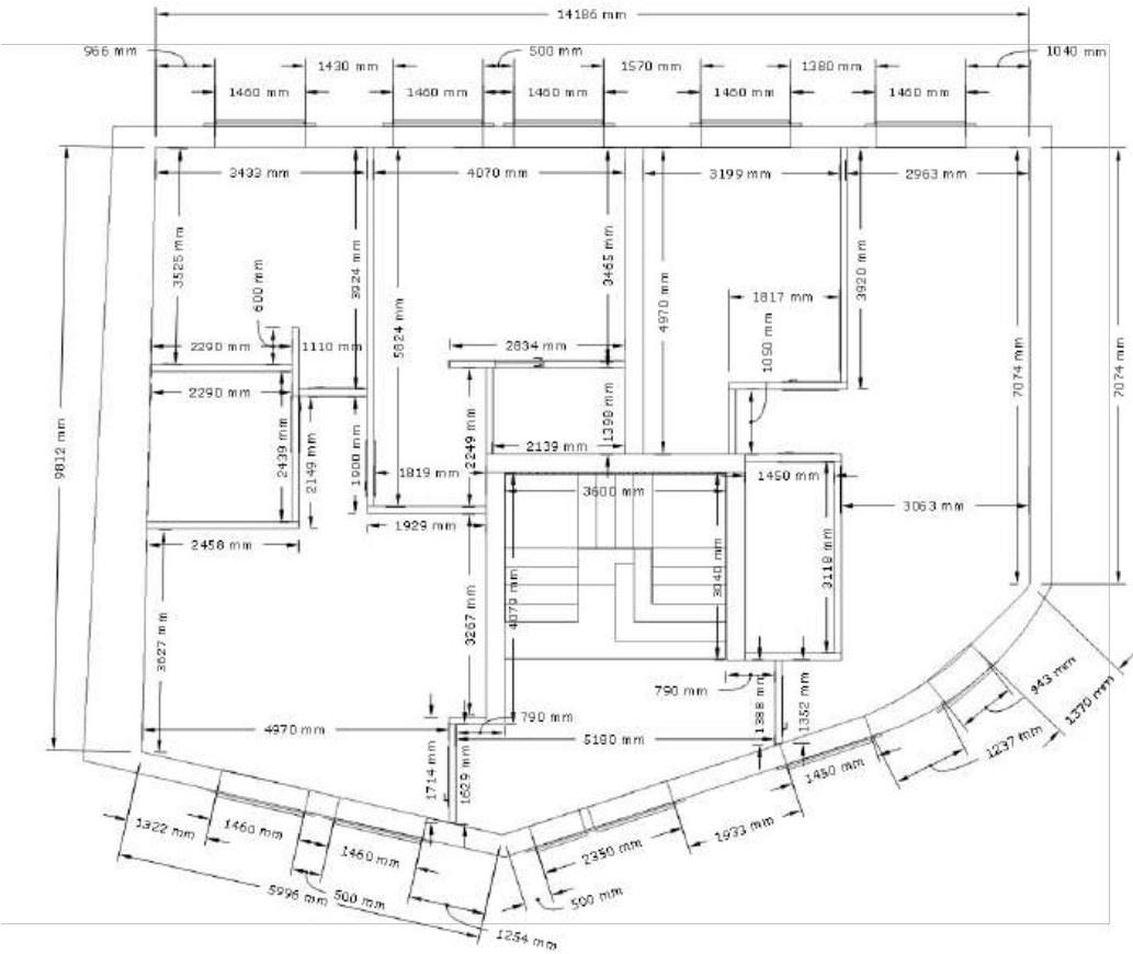
PLANTA COTADA PISO 0
